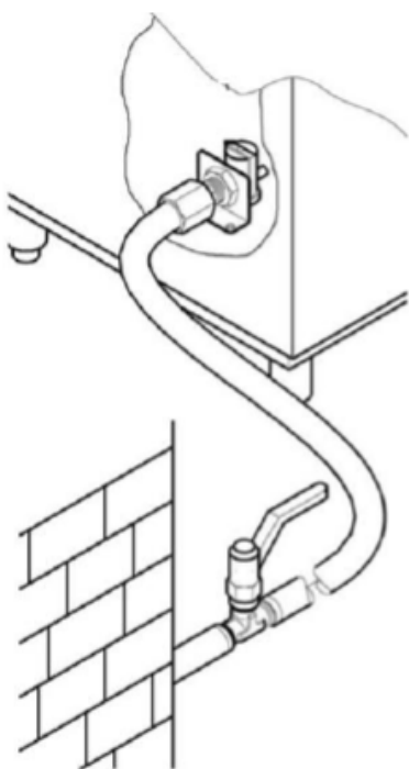
Připojení k vodovodní síti
